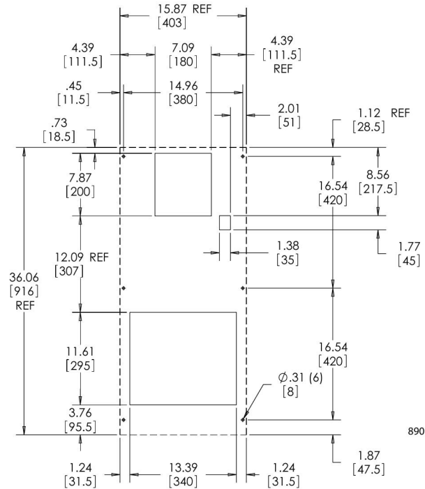
CUTOUT DIMENSIONS
